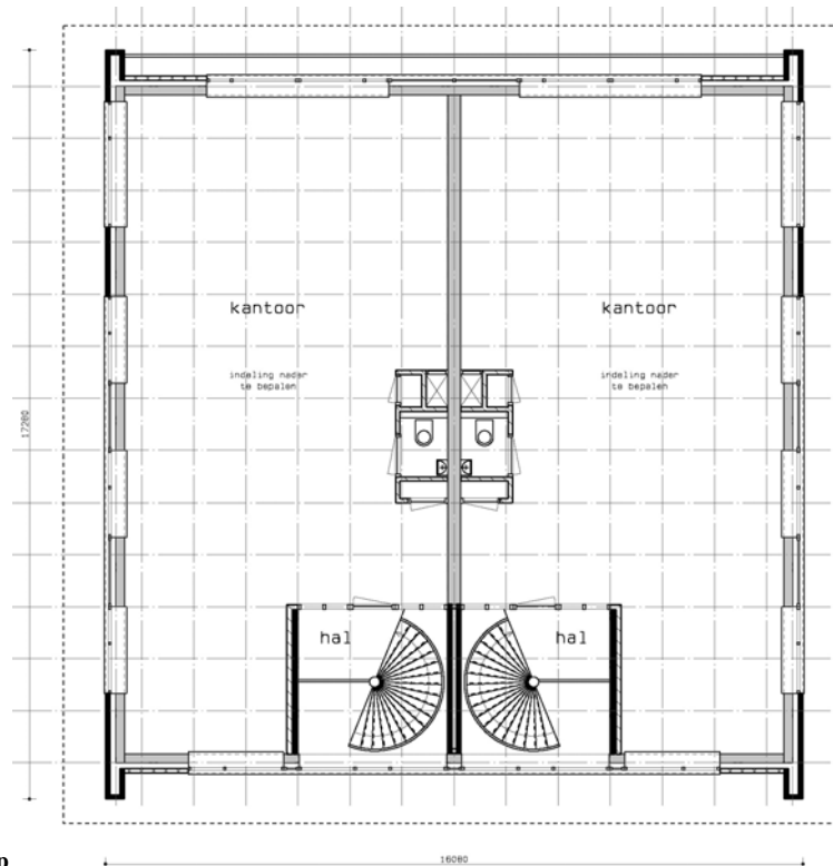
1e verdieping 2/1 kap
