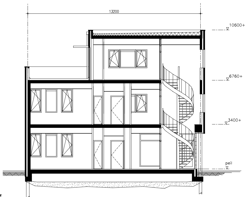
Doorsnede Poortgebouw
