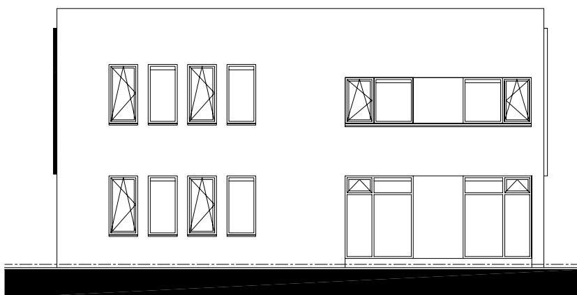
Achtergevel 2/1 kap
