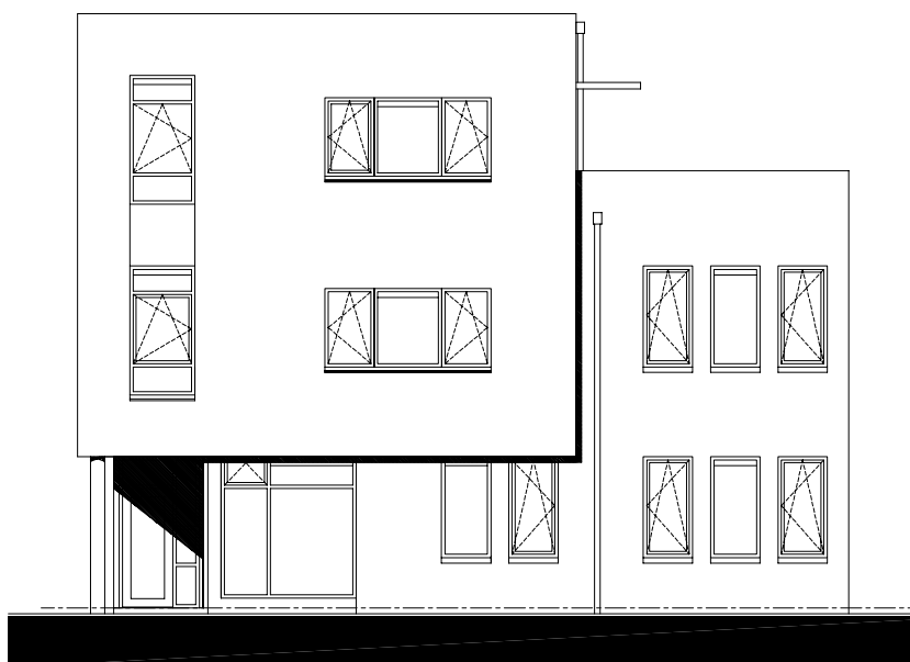
Zijgevel Poortgebouw
