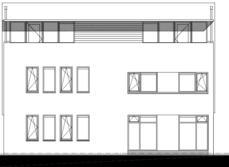
Achtergevel Poortgevel
