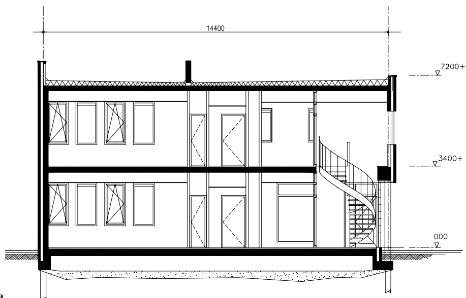
Doorsnede villa
