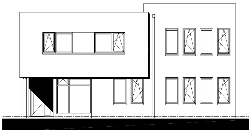
Zijgevel 2/1 kap
