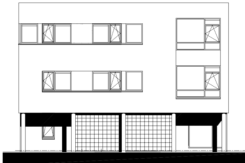
Voorgevel Poortgebouw
