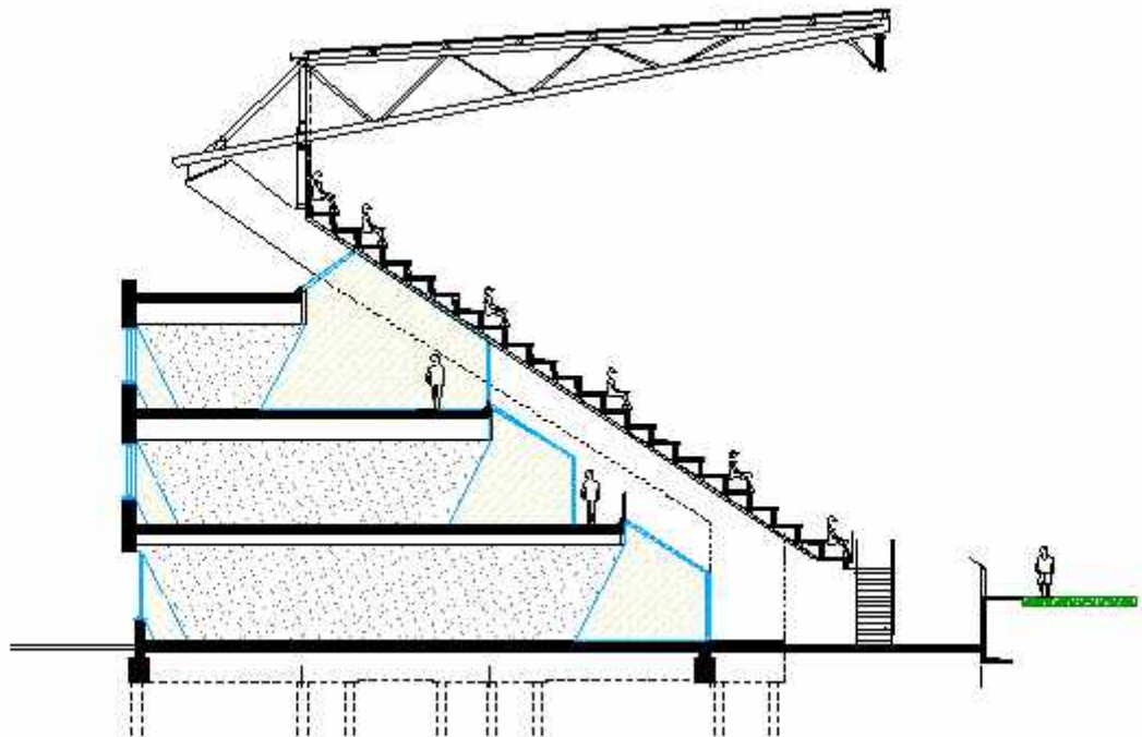
DWARSDOORSNEDE C
